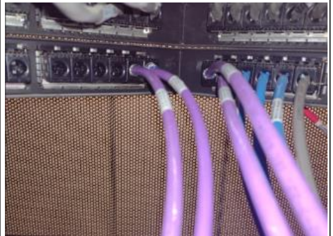
Ponchado y marquillado en patch panel
